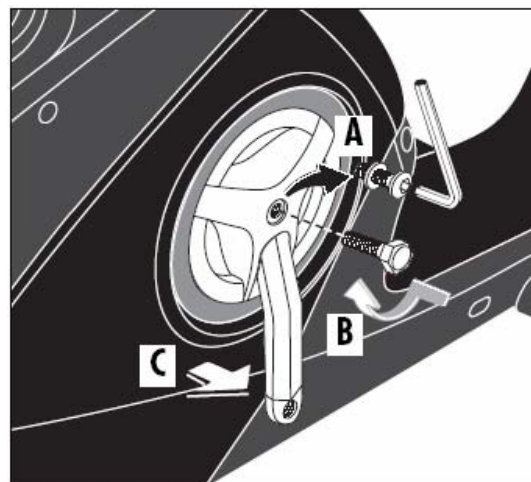
Демонтаж шатуна
